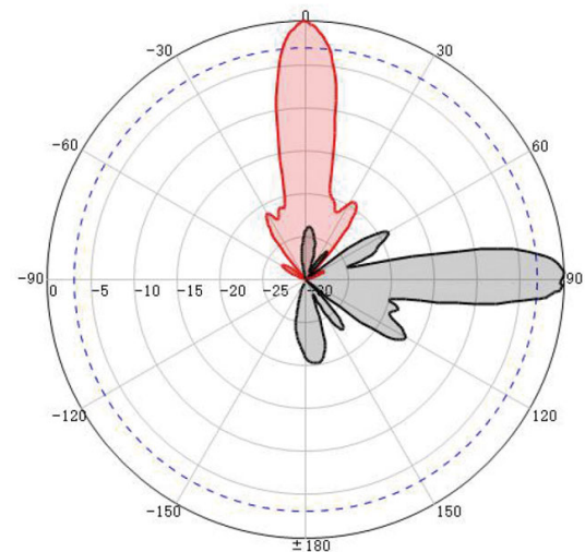
V-Pol@2700MHz
