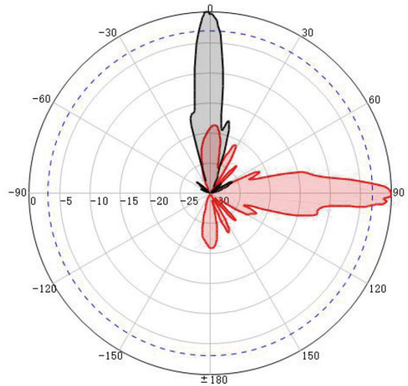
V-Pol@3500MHz
