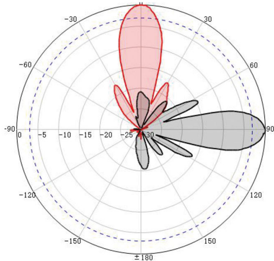
H-Pol@1710MHz
