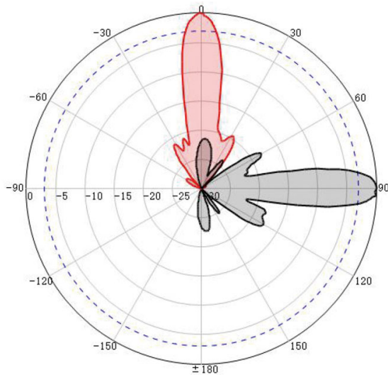
H-Pol@2700MHz
