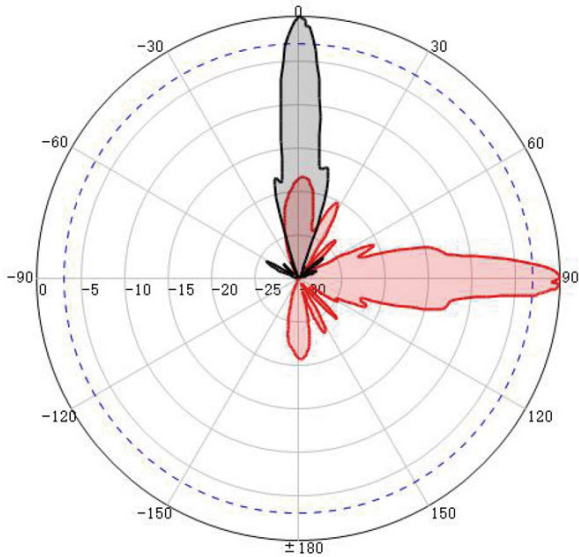
H-Pol@3500MHz
