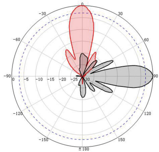
V-Pol@1710MHz
